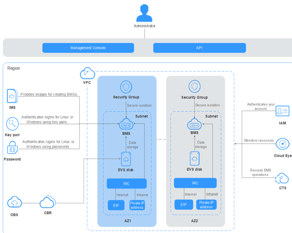
Figura 2-1 Arquitectura del sistema
