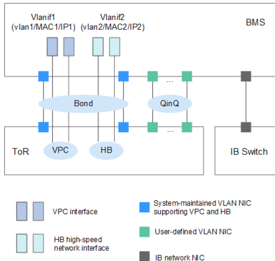
Figura 8-1 Redes de BMS
